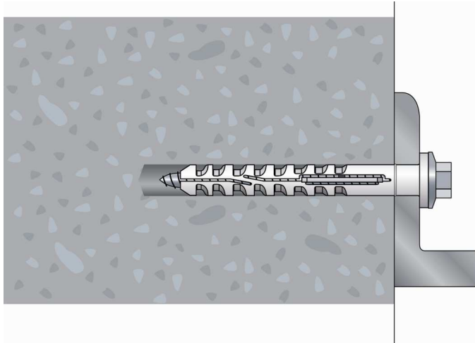
Abb. 3: Verarbeitung in Beton
