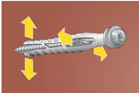
Abb. 4: 4-fach-Spreizung sorgt für sicheren Halt in jedem Mauerwerk
