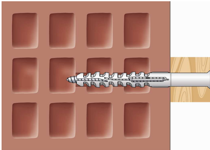
Abb. 2: Verarbeitung im Mauerwerk
