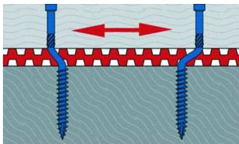
Abb. 3: Durch den Einsatz der Terrassenbauleiste wird ein Abstand zwischen Unterkonstruktion und Diele geschaffen. Aus der Scher- wird eine Biegebelastung, die von den Schrauben problemlos ausgehalten wird.
